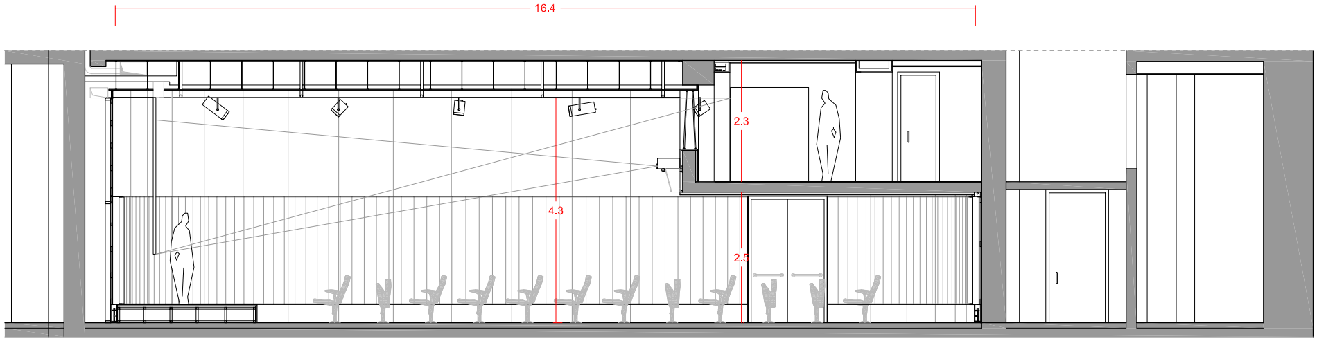
Secció AA'
